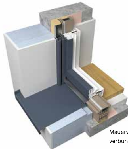
monolithisches Mauerwerk
