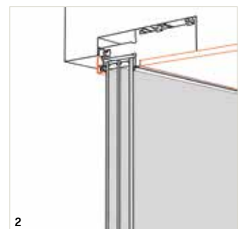
innen rahmenloser Einbau
