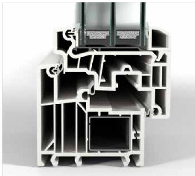
Schnitt durch einen Finstral-Kunststoff-Rahmen: FIN-Window Slim-line 77 Kunststoff-Kunststoff
