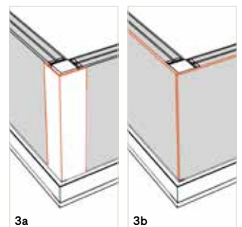
mit Glas um die Ecke
