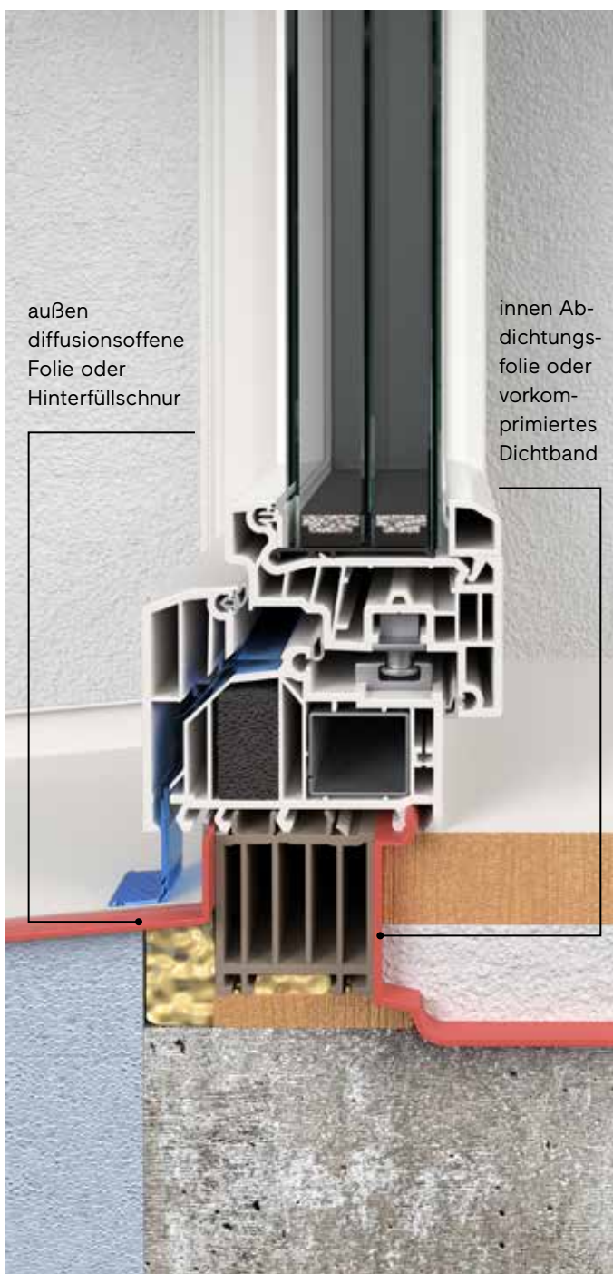
Einstufige Montage direkt auf Mauer
